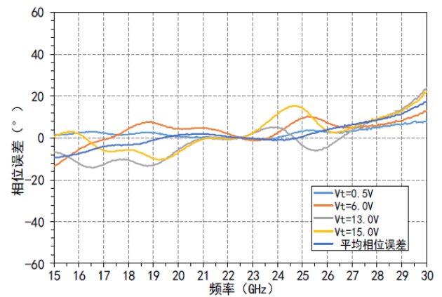
相位误差VS频率@Pin=-10dBm
