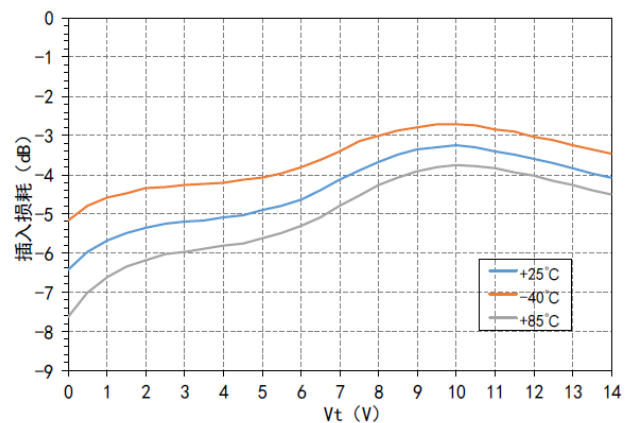
插入损耗VS Vt@22GHz
