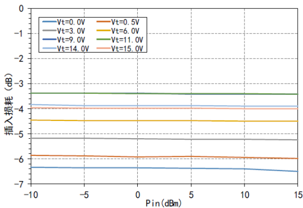
插入损耗VS Pin@22GHz
